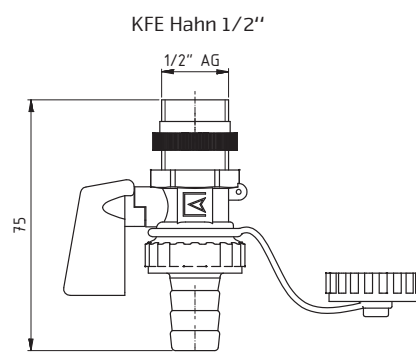
Entlüftungsstopfen 1/2"
