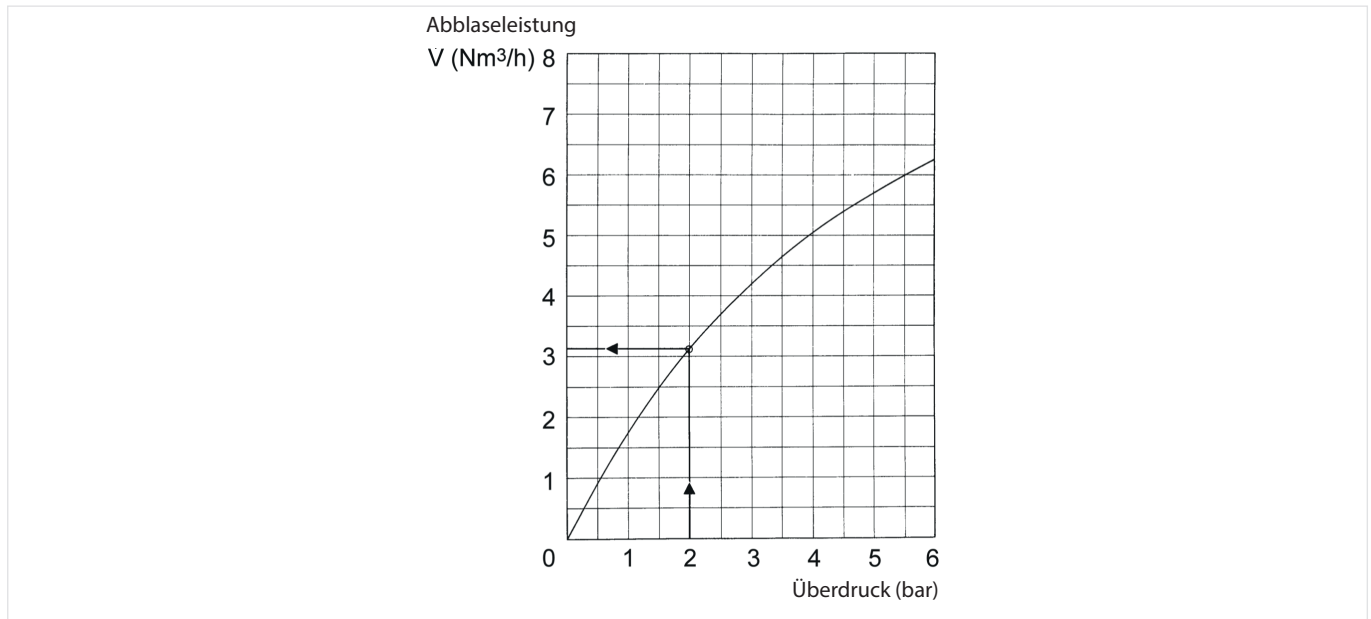
Abb. 1 Abblaseleistung
