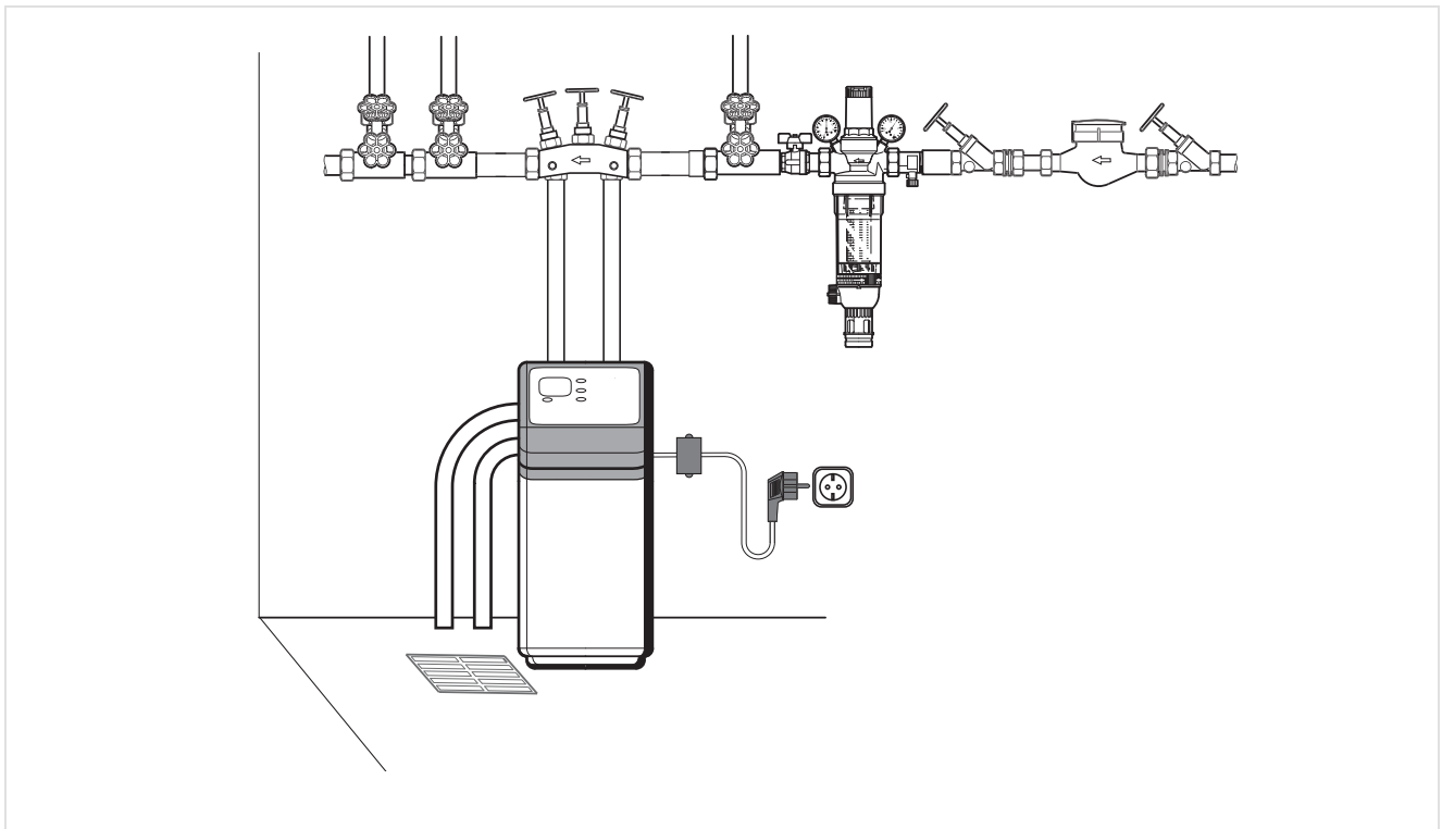
Abb. 1 Standard Installationsbeispiel für das Enthärtungsgerät KaltecSoft KS10S
