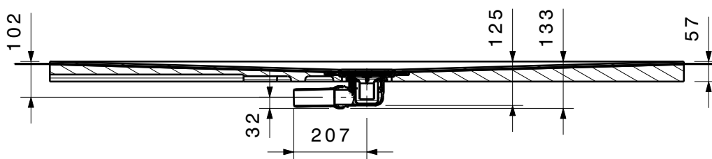
Schnitt B-B
