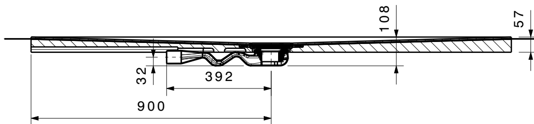
Schnitt A-A
