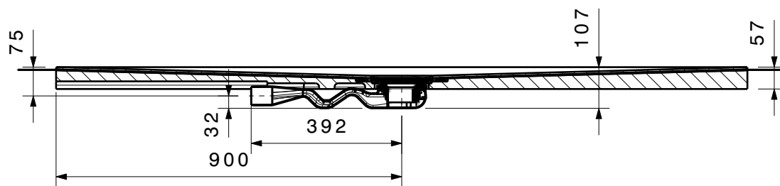
Schnitt A-A
