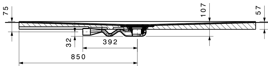
Schnitt A-A
