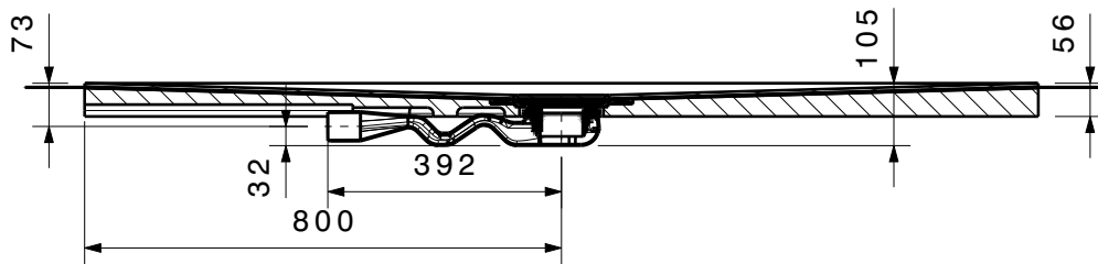
Schnitt A-A
