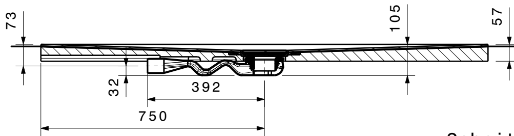
Schnitt A-A
