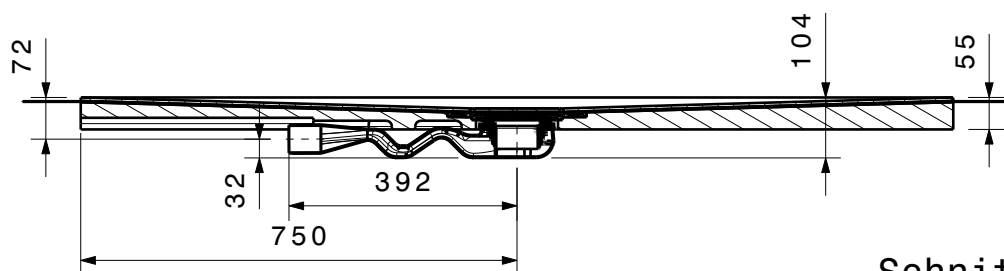
Schnitt A-A
