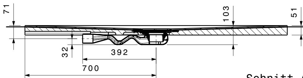
Schnitt A-A
