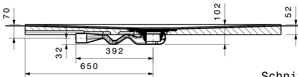
Schnitt A-A
