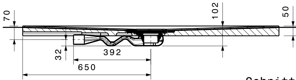
Schnitt A-A
