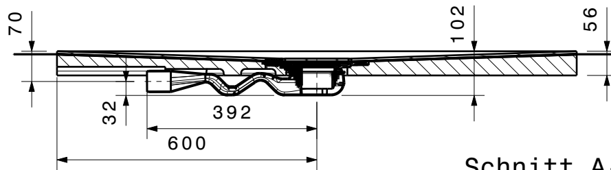
Schnitt A-A
