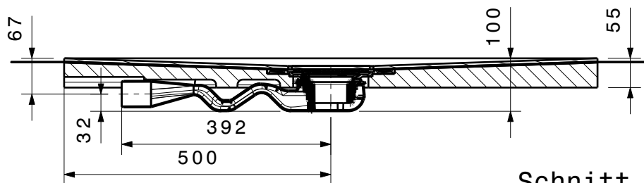
Schnitt A-A
