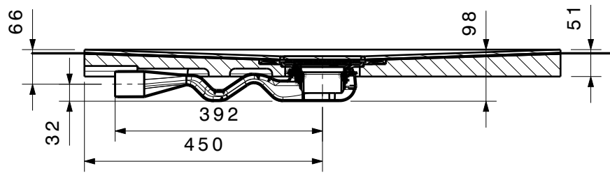
Schnitt A-A
