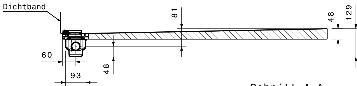
Schnitt A-A
