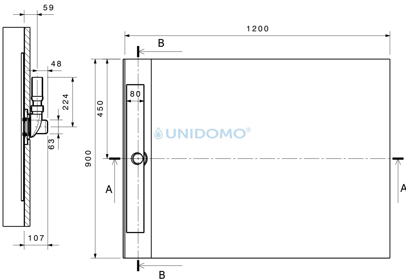
Schnitt B-B
