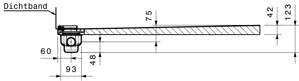
Schnitt A-A
