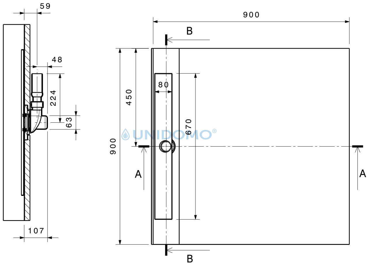
Schnitt B-B
