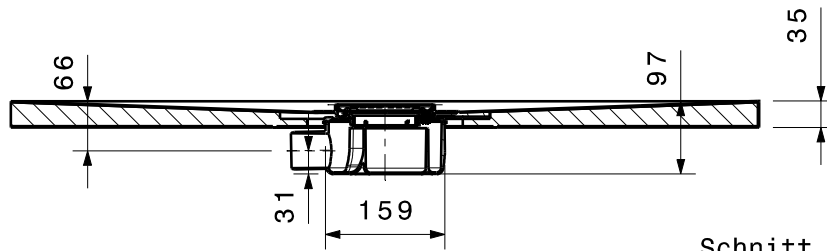
Schnitt A-A
