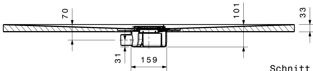
Schnitt A-A
