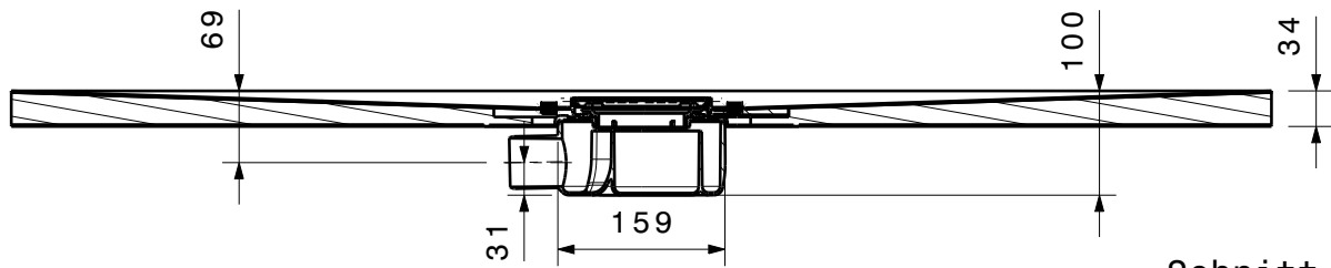
Schnitt A-A
