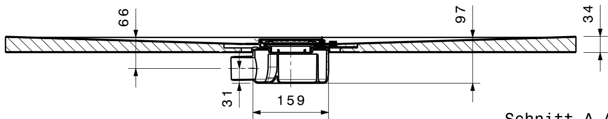
Schnitt A-A
