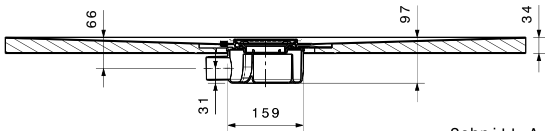
Schnitt A-A
