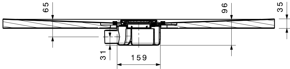
Schnitt A-A
