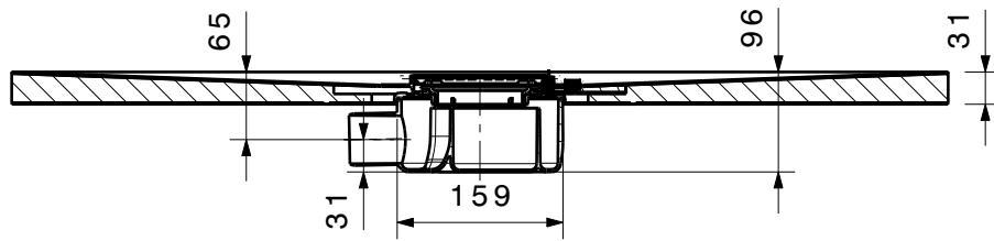
Schnitt A-A
