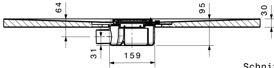
Schnitt A-A
