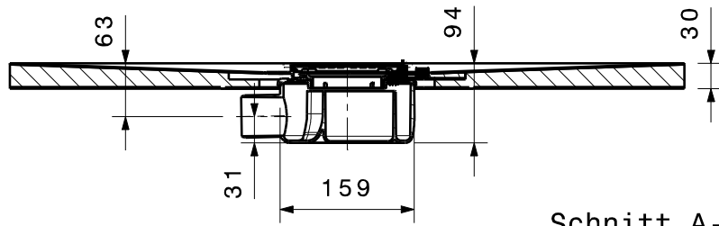
Schnitt A-A
