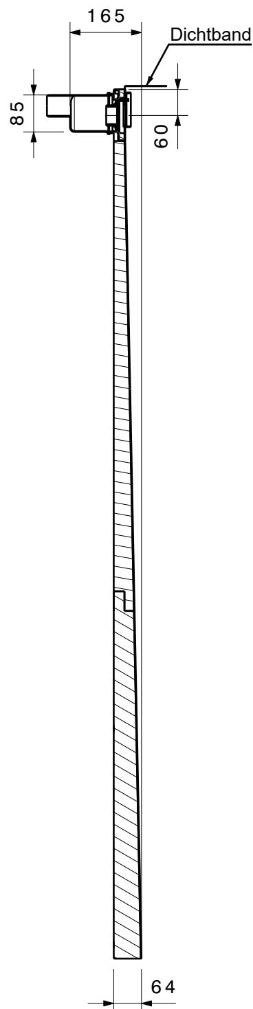
Schnitt A-A
