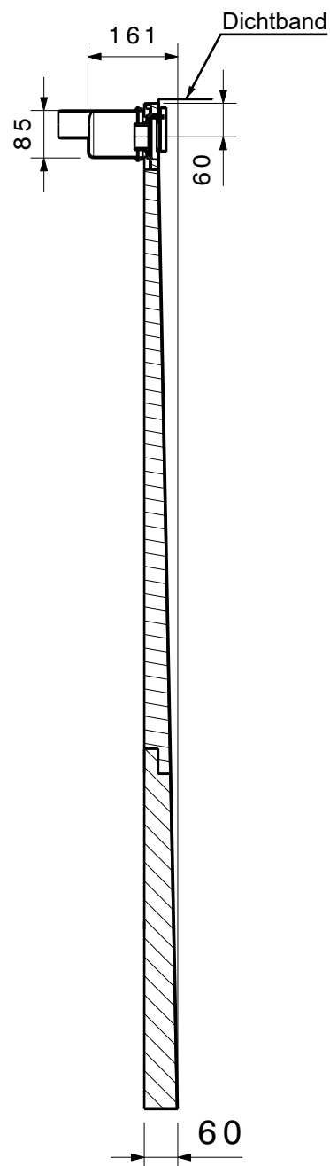
Schnitt A-A
