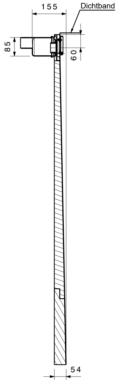
Schnitt A-A
