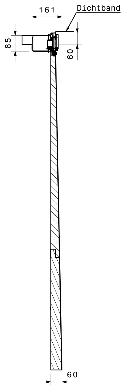
Schnitt A-A
