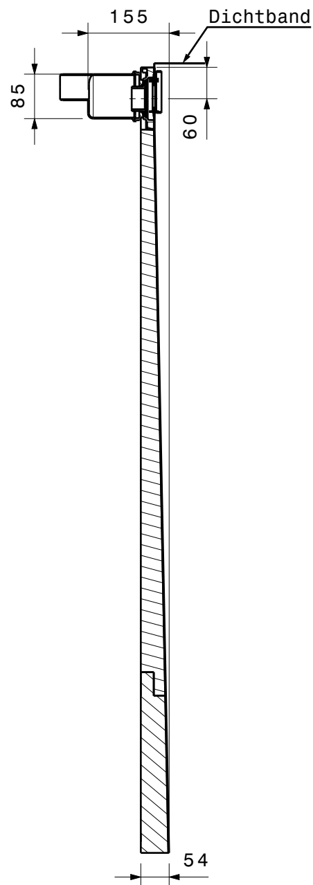
Schnitt A-A
