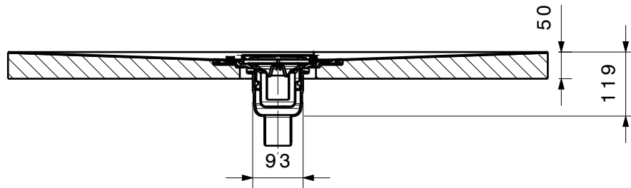
Schnittansicht A-A (2)
