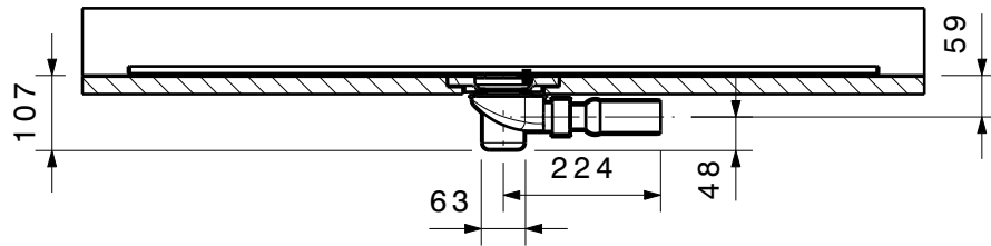
Schnitt B-B
