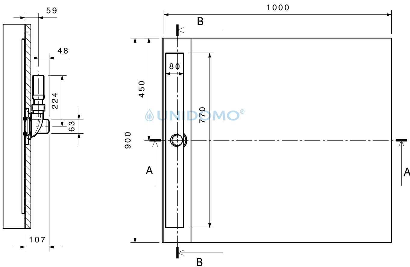
Schnitt B-B
