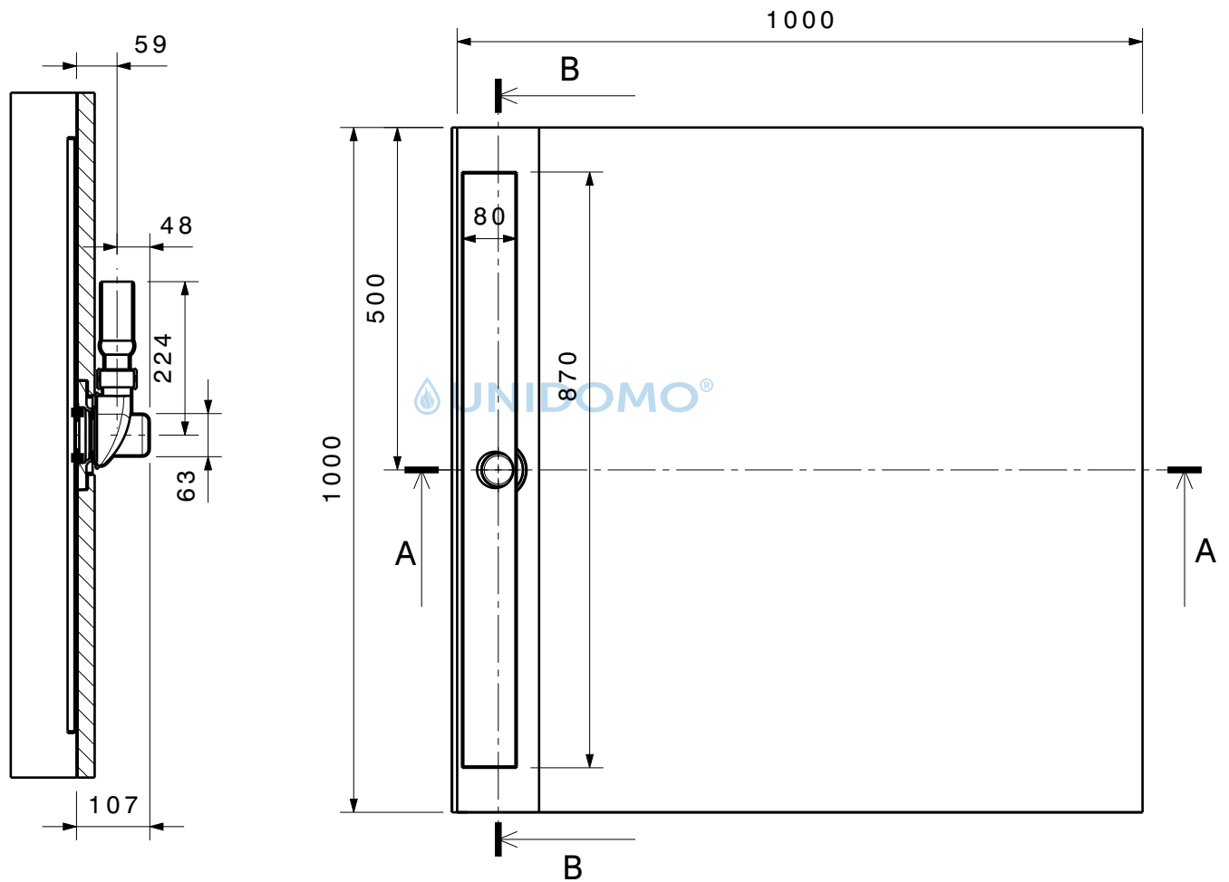
Schnitt B-B
