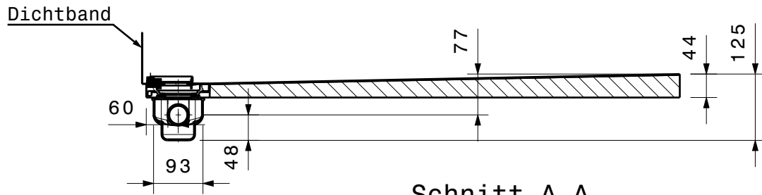
Schnitt A-A
