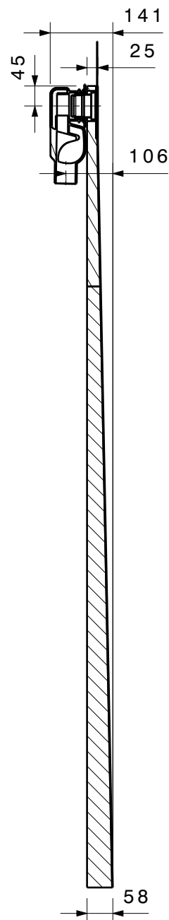
Schnitt B-B
