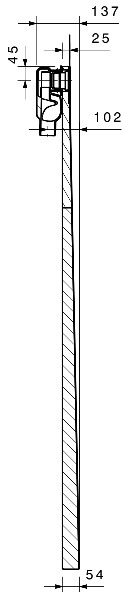
Schnitt B-B
