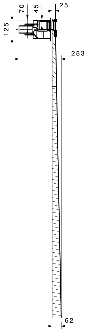
Schnitt C-C
