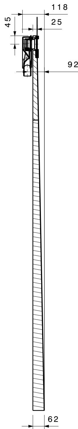
Schnitt A-A
