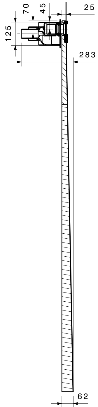
Schnitt C-C
