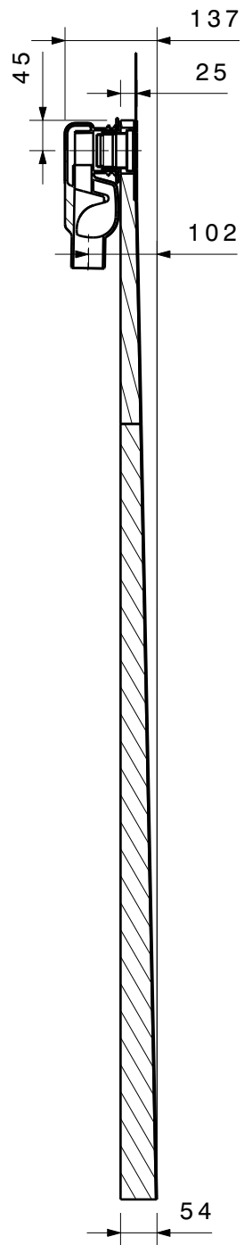
Schnitt B-B
