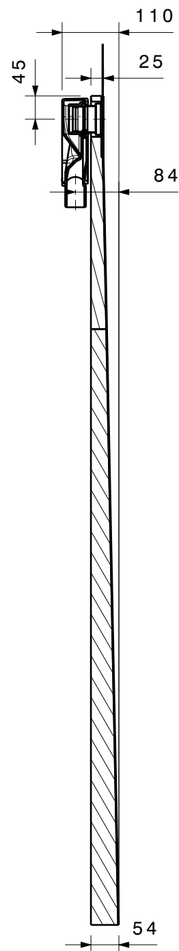
Schnitt A-A
