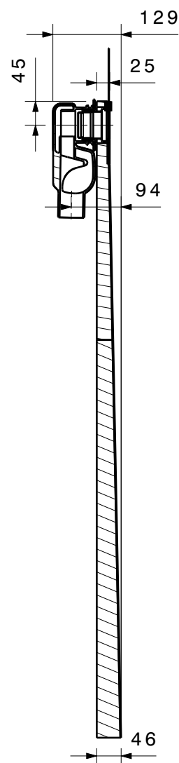
Schnitt B-B
