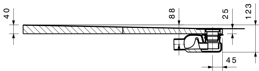
Schnitt B-B
