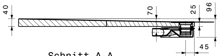
Schnitt A-A
