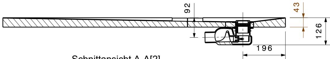
Schnittansicht A-A[2]
