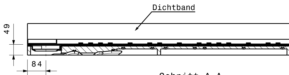
Schnitt A-A
