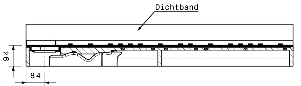
Schnitt A-A
