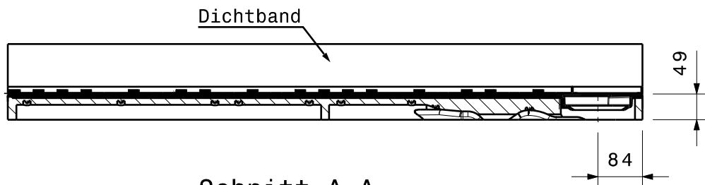
Schnitt A-A
